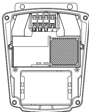
Fig. 10 Protection module
