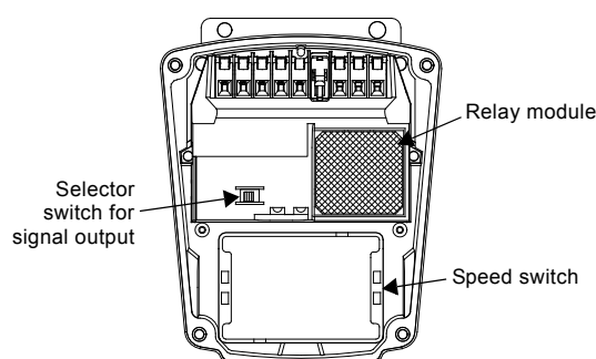
Fig. 11 Relay module
