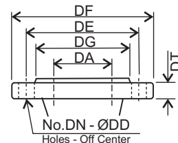
Discharge Flange (JIS 10kgf/cm 2 )
